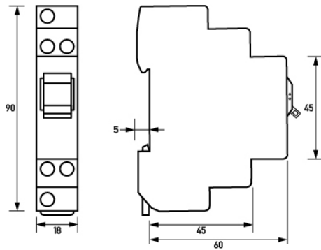
Maßzeichnung Gruppenansicht
