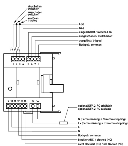
Anschlusschema
