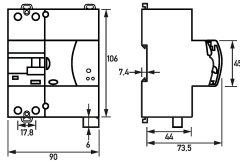
Maßzeichnung Gruppenansicht
