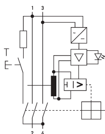
Schaltungsbeispiel Fehlerstromschutzschalter DFS 2 040-2/0,30-B SK
