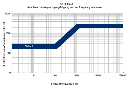
Diagramme Fehlerstromschutzschalter DFS 2 040-2/0,30-B SK
