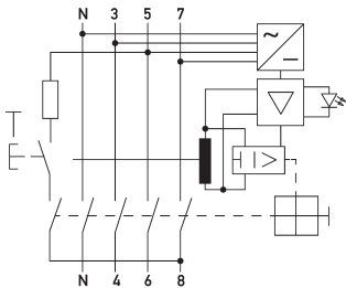
Anschlussschema
