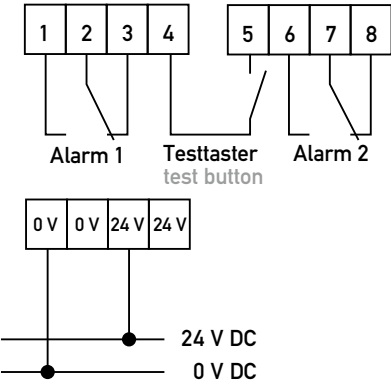
▲ Anschlusschema der Alarmkontakte
