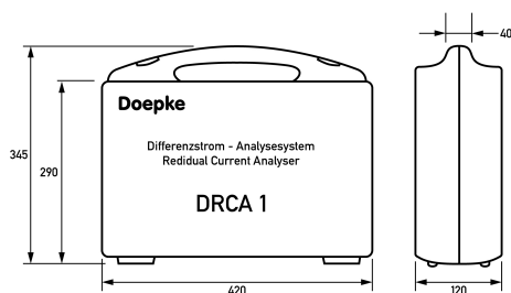
Maßzeichnung Gruppenansicht
