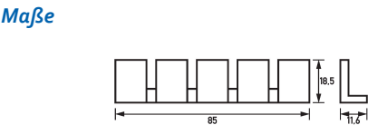
Maßzeichnung Berührungsschutzkappen EV-S BS
