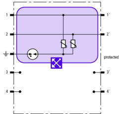
Prinzipschaltbild BXT ML2 MY 250
