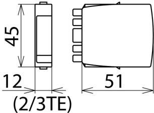
Maßbild BXT ML2 MY 250
