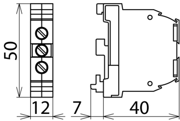
Maßbild SLK 16
