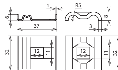
Maßbild
