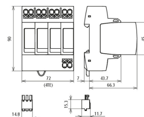
Maßbild DG MP TT 320 FM
