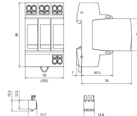
Maßbild DG MP TNC ACI 275 FM
