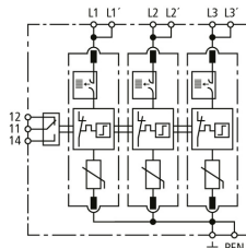
Prinzipschaltbild DG MP TNC ACI 275 FM
