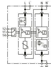
Prinzipschaltbild DG MP TT 2P ACI 385 FM
