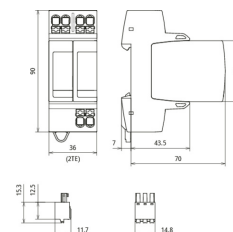
Maßbild DG MP TT 2P ACI 275 FM
