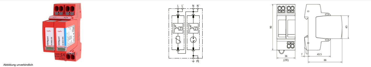
Abbildung unverbindlich Prinzipialschaltbild DG MP TT 2P 275 Maßbild DG MP TT 2P 275
