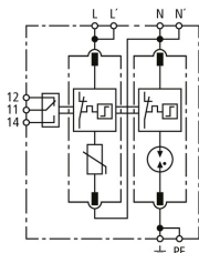
Principalschaltbild DG MP TT 2P 275 FM
