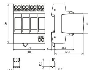
Maßbild DG MP TT 150 FM
