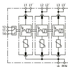
Prinzipschaltbild DG MP TNC 440 FM
