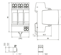
Maßbild DG MP TNC 440 FM
