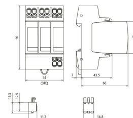
Maßbild DG MP TNC 385 FM
