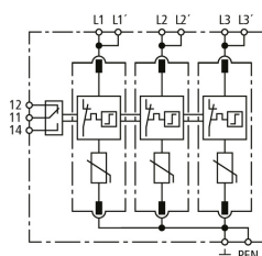
Prinzipialschaltbild DG MP TNC 385 FM
