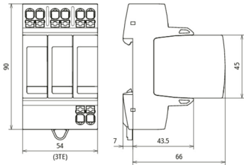
Maßbild DG MP TNC 275 FM
