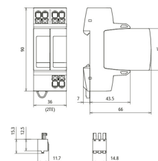
Maßbild DG MP TN 275 FM
