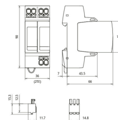
Maßbild DG MP TN 150 FM
