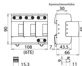
Maßbild DV M TNC 255 FM
