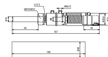
Maßbild
