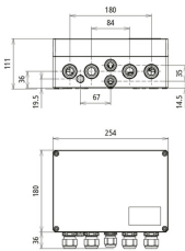
Maßbild DCU 2 YPV 1+2 1000 2M 2S FM
