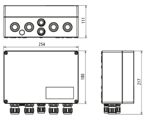
Maßbild DCU 2 YPV 1100 2M 2S
