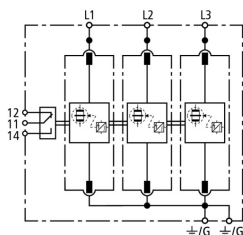
Prinzipschaltbild DB MU 3PY 480 3W+G R
