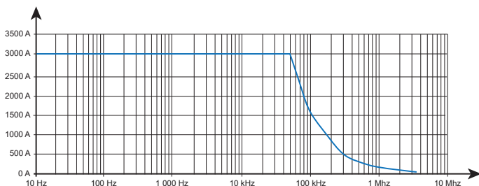
Portata 3000 A
