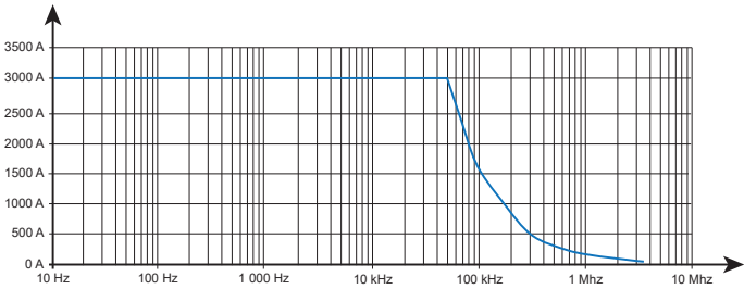
Messbereich 3000 A
