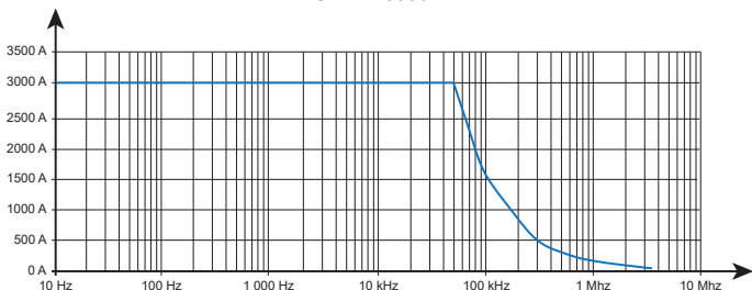
Calibre 3000A
