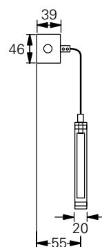
Wandparallele Montage mit Seilabhängung
