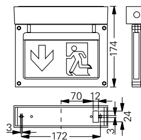
Deckenaufbau
