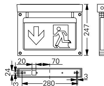
Deckenaufbau
