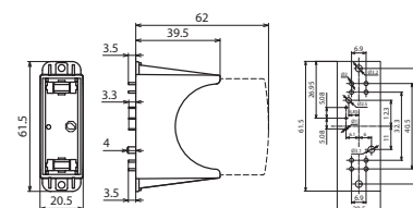
Maßbild
