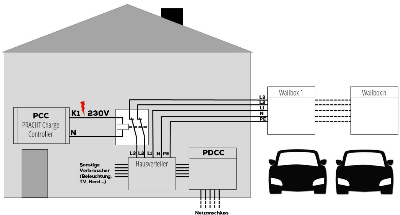
Abbildung 6 Beispiel: Phasenabwurf-Schaltung
