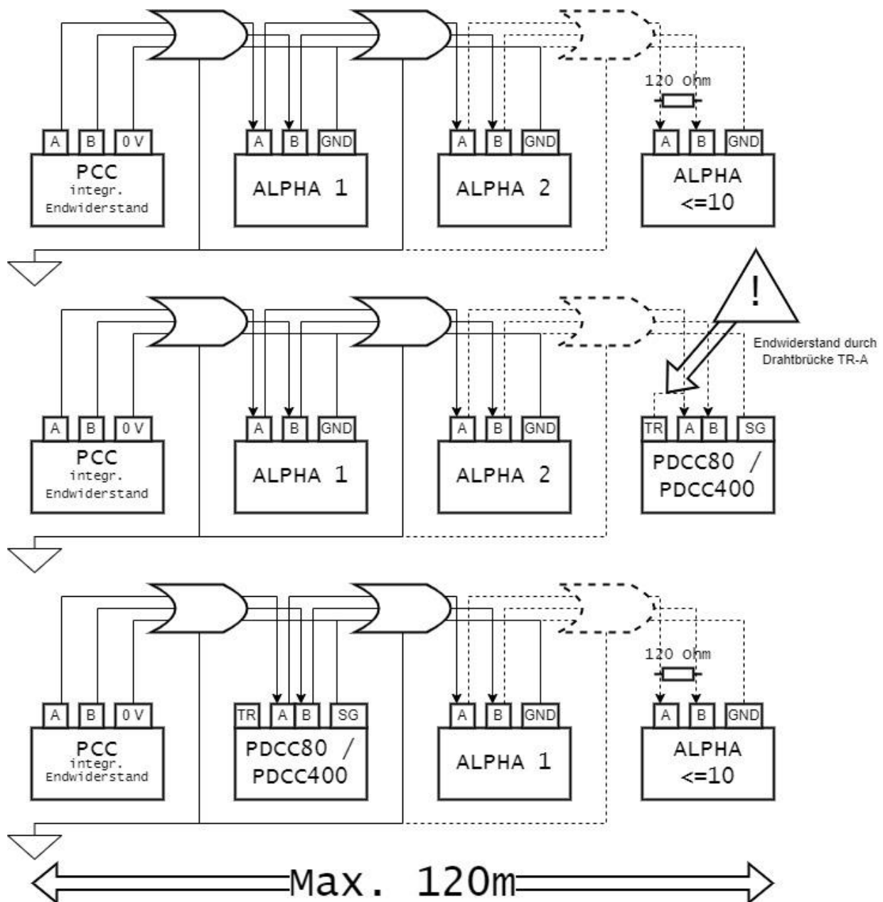
Abbildung 3 Modbus-Verkabelung
