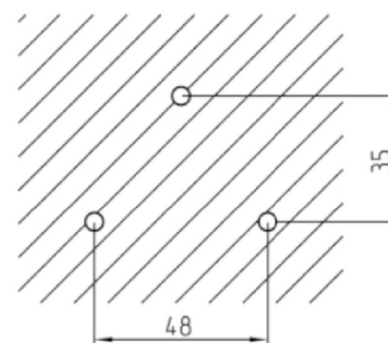
Bohrbild
