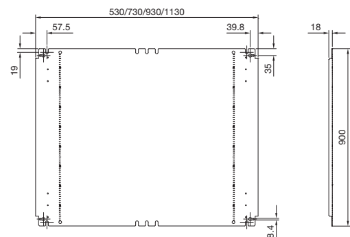
Montageplatte
