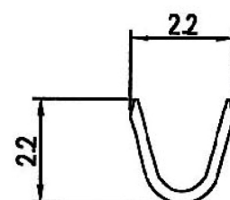
A-A SECTION
