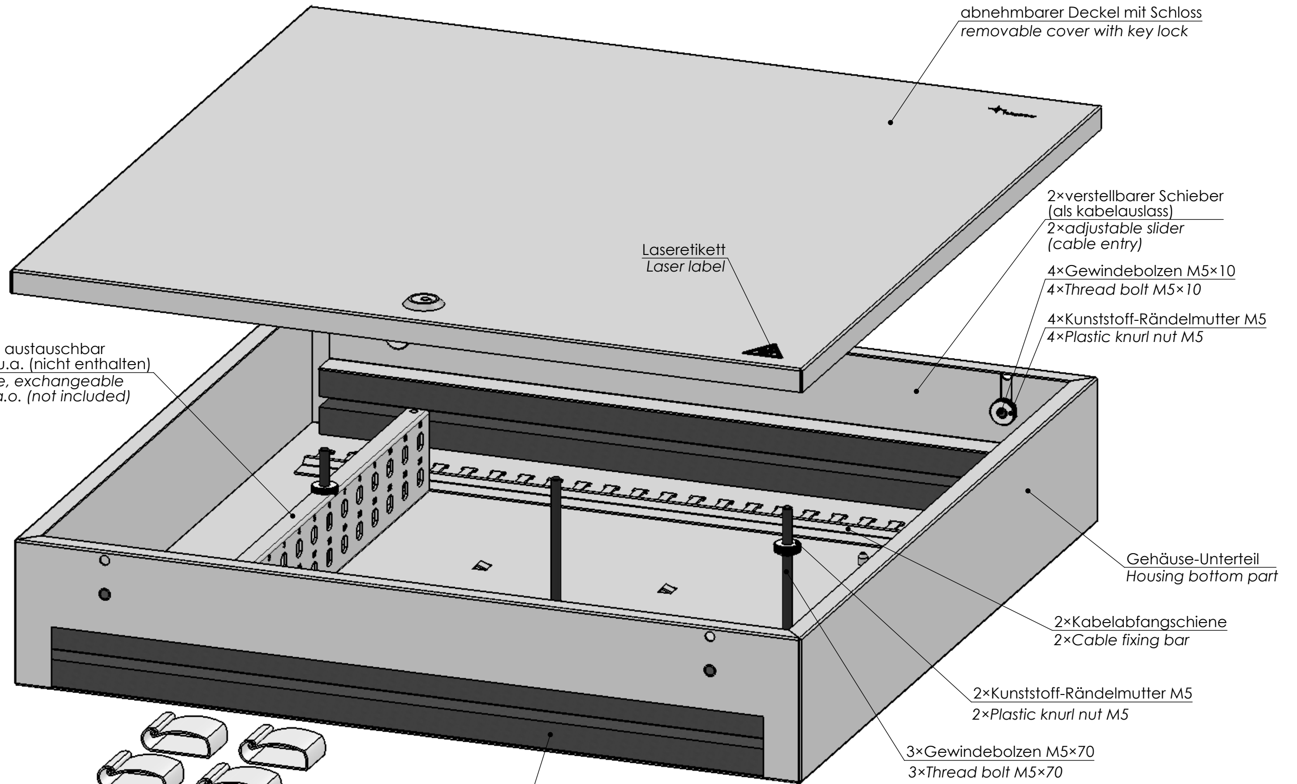
Kabelschellen-Set beigelegt Cable clamps set arranged
