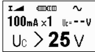
Bild 3.6 Berührungsspannung > 25 V
