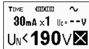
Bild 3.1 Anzeige von (Fremd-) Spannung < 190 V
