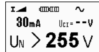
Bild 3.2 Anzeige von (Fremd-) Spannung > 255 V
