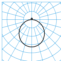
Solegra WD1 OTA 2600-830 + WD1 ZP 01 TX062729 UGR I = 22.2 UGR q = 22.2 DIN 5040: A40 UTE: 0,95 E + 0,05 T CEN Flux Code: 46 78 95 95 100 45 77 94 5 ■ C0 - C180 ■ C90 - C270
