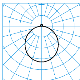
Solegra WD1 OTA 2600-830 + WD1 ZP 05 TX062772 UGR I = 22.2 UGR q = 22.2 DIN 5040: A40 UTE: 0,95 E + 0,05 T CEN Flux Code: 46 78 95 95 100 45 77 94 5 ■ C0 - C180 ■ C90 - C270
