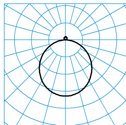
Solegra WD1 OTA 2600-830 + WD1 ZP 03 TX062771 UGR I = 22.2 UGR q = 22.2 DIN 5040: A40 UTE: 0,95 E + 0,05 T CEN Flux Code: 46 78 95 95 100 45 77 94 5 ■ C0 - C180 ■ C90 - C270
