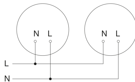
Schaltplan Master-Master Vernetzung
