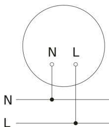
Schaltplan Slave / Funk-Master Vernetzung
