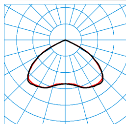
7650IP L-SHB 230V Inotec L37 03 TX277167
