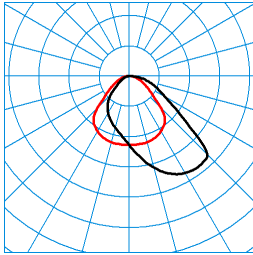
Cultega T COM PAW 600-930 KL 05 TX280846
