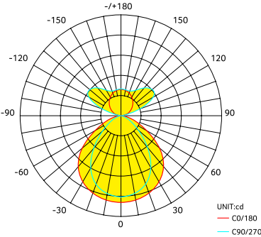
indirektes / direktes Licht
