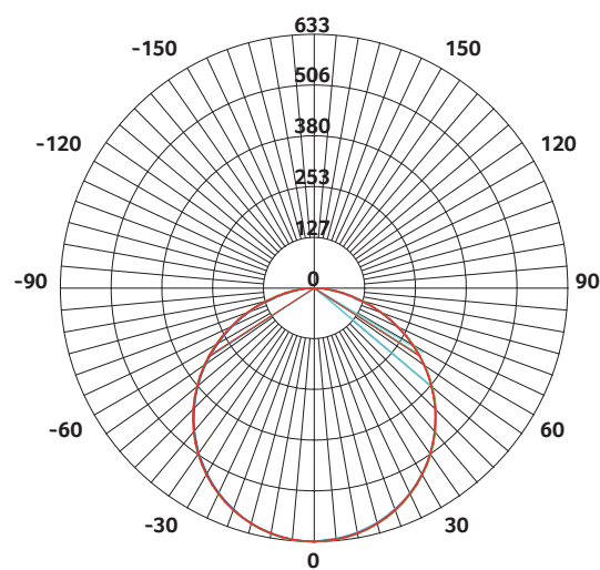
Lichtverteilung
