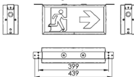
Deckenmontage mit Winkel außen
