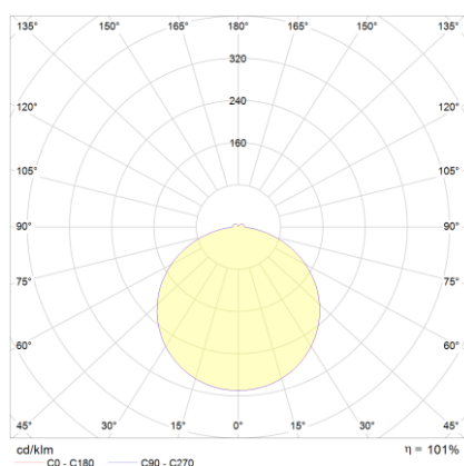
Lichtverteilungskurve
