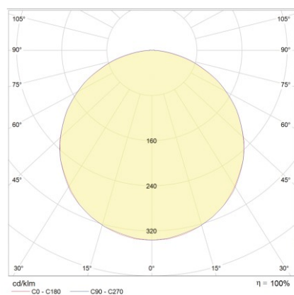
Lichtverteilungskurve
