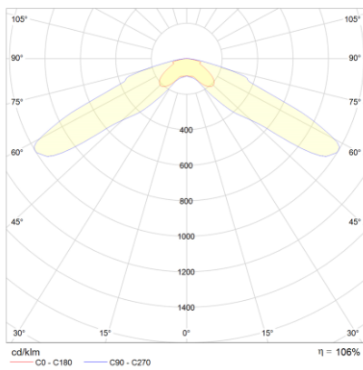
Lichtverteilungskurve
