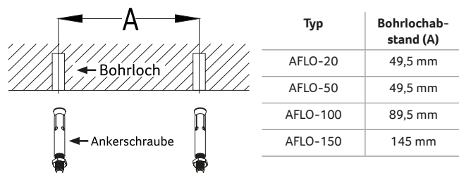
Abb. 4: Bohrlochabstände
