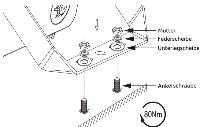
Abb. 5: Leuchte befestigen
