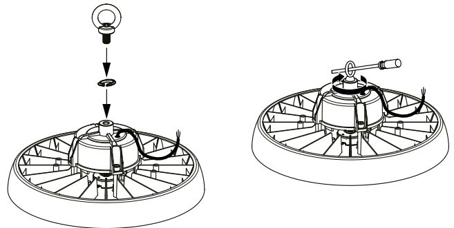
Abb. 3: Gewindeöse einschrauben
