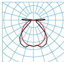
OleveonF B 1500 8000-865 PC TX056220
